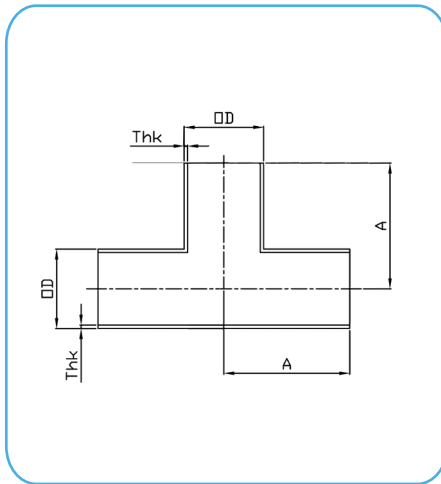
7WWW-TEE BW x BW ASME BPE DT-4.1.2-1
