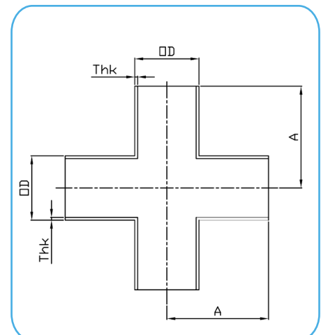
9WWW-CROSS BW x BW ASME BPE DT-4.1.2-1
